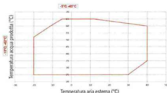
Fig. 4 - Campo di lavoro pompa di calore ad alta temperatura
