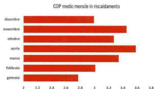
Fig. 6 - COP medio mensile in riscaldamento località Verona per PDC alta temperatura
