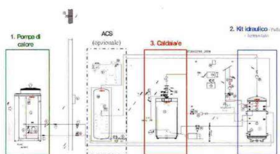
Fig. 2 - Schema tipico di un sistema ibrido commerciale
