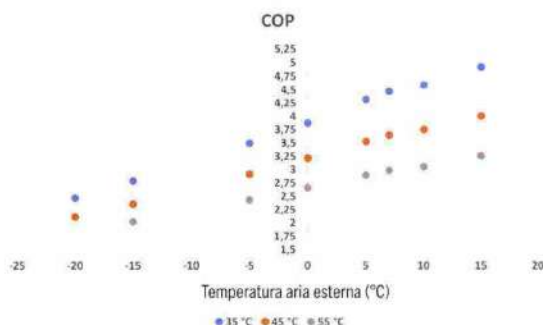
Fig. 5 - Andamento COP per diverse temperature di mandata al variare della temperatura aria esterna
