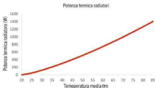
Fig. 1 - Esempio di curva di potenza termica di un radiatore ( P_{nom}=1\text{ kW} , n=1,3 , \theta_{amb}=20\text{ °C} )
