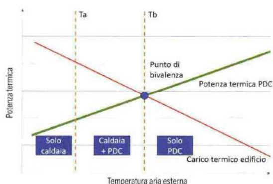
Fig. 3 - Schema delle configurazioni operative del sistema ibrido in funzione della regolazione
