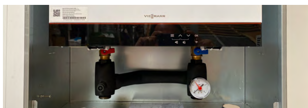
Collettore ibrido installato all'interno del box (sistema Vitodens 100-E Hybrid)
