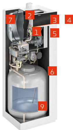
Vitodens 222-F Con bollitore smaltato ad accumulo (modello B2TF)
