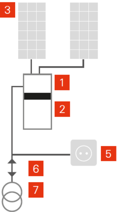
Impianto fotovoltaico con accumulo (sistema ibrido)
